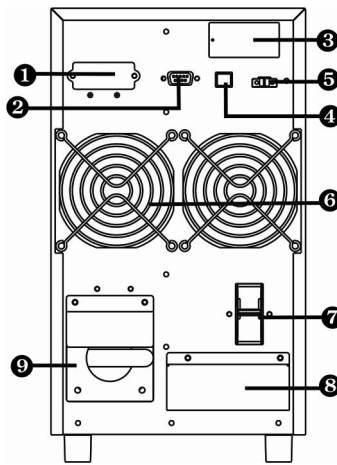
图 2: 6KL/10KL 背面面板
